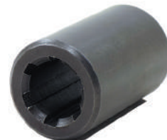
Luva 06 Estrias Diâmetro Int.: 26,20mm
