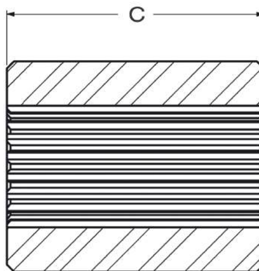
SEÇÃO C-C
