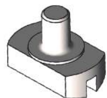
Porta Retentor Diâmetro Ext.: 217,00mm Diâmetro Int.: 168,00mm Espessura: 12,50mm
