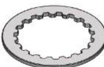
Arruela Diâmetro Ext.: 94,00mm Diâmetro Int.: 73,0/66,2mm Espessura: 3,80 19 Dentes Interno
